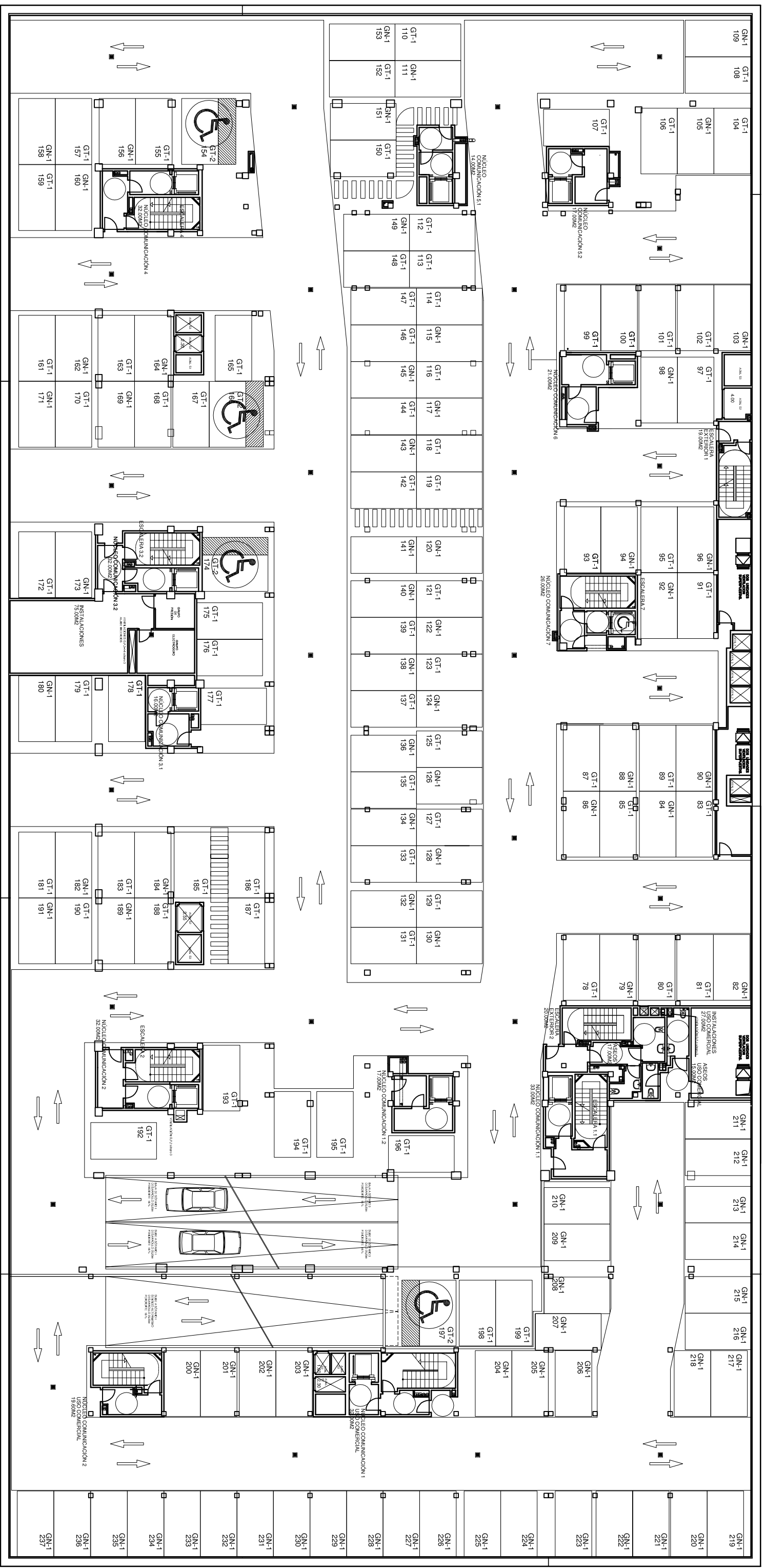
PLANTA SÓTANO 2
